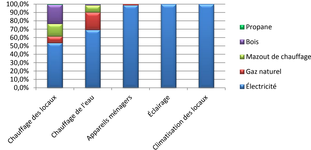
Figure 21: Pourcentage de consommation par type d'énergie pour chacune des utilisations finales de l'énergie du secteur résidentiel, Québec (2009) Source : OEE. 2012
