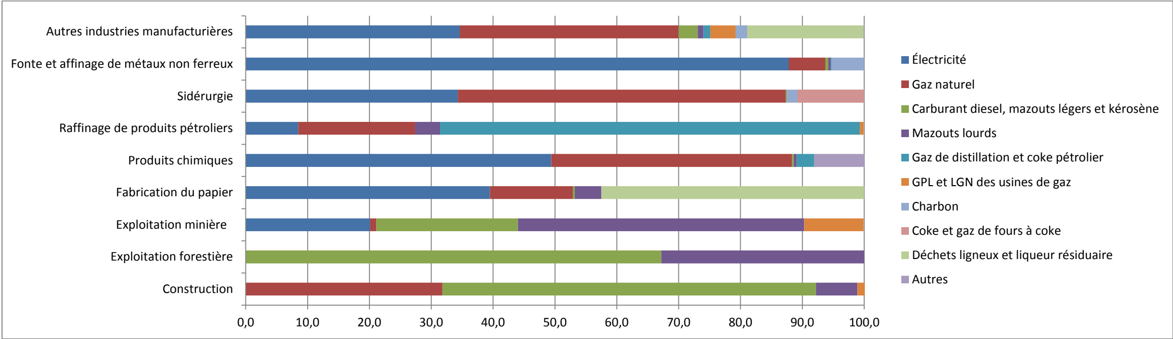
Figure 34 : Pourcentage de consommation par ressource énergétique pour le secteur industriel, Québec (2009)
