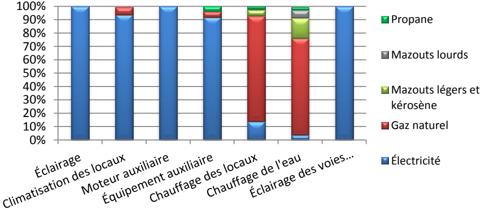
Figure 30 : Pourcentage de consommation par type d'énergie pour chacune des utilisations finales de l'énergie du secteur commercial et institutionnel, Québec (2009) Source : OEE 2013a; compilation CRE Laurentides
