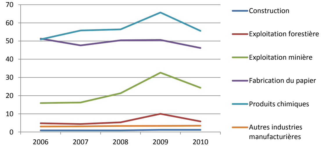
Figure 35 : Évolution de l'intensité énergétique (MJ/PIB-2002$) pour les secteurs industriels à l'étude, Québec Source : OEE. 2013b
