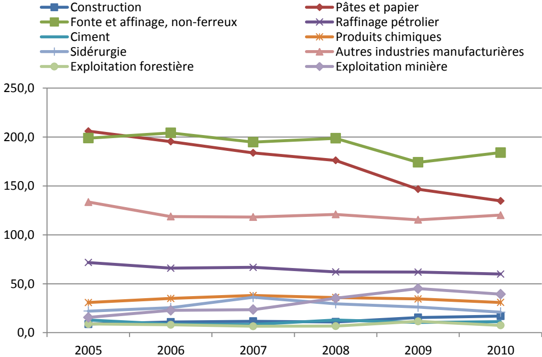
Figure 32 : Évolution de la consommation d'énergie (PJ) dans le secteur industriel, Québec Source : OEE, 2013b
